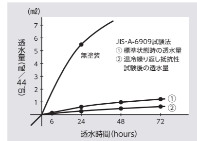
[グラフ1] 浸透型吸水防止剤 ボンガード 透水性試験結果
