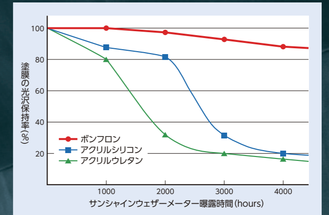
ボンフロンAC#1100(#1500)SR上塗の促進耐候性試験
