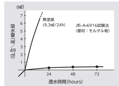
[グラフ2] 浸透型吸水防止剤 ボンガード 吸水性試験結果
